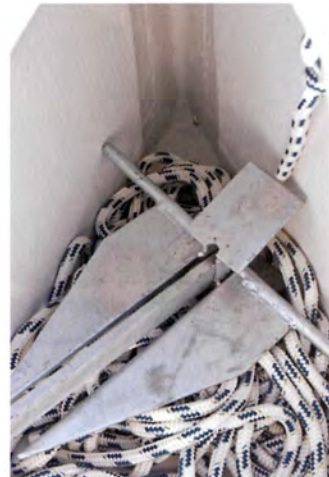
Ankerkasten mit Entwässerung an der tiefsten Stelle.
